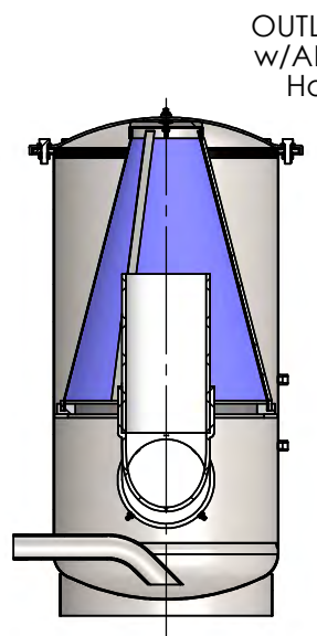
SECTION A-A
